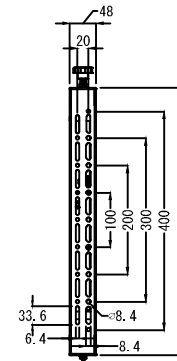
収納時奥行 前後アジャスター範囲 ±7mm
