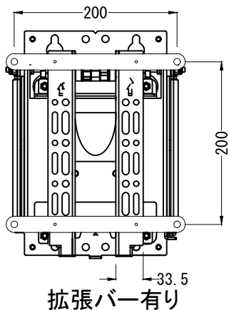
VESA金具 上方向調節範囲 +12mm
